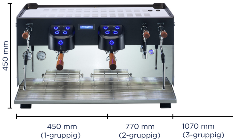
Frontansicht
